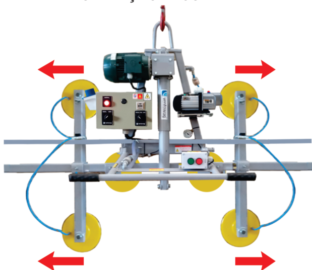
OPERAÇÃO RECOLHIDA
